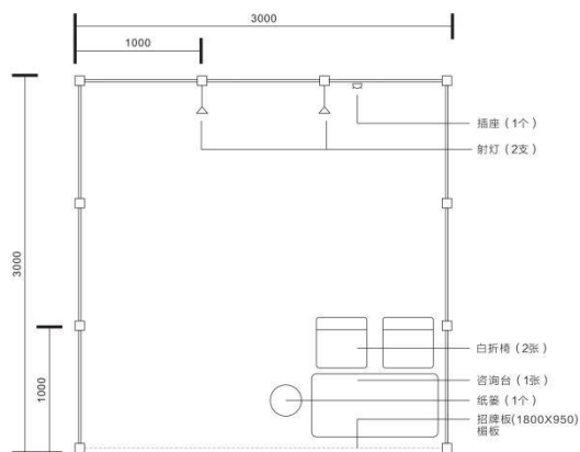
平面示意图
